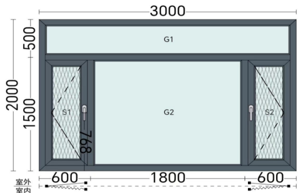
部分实验室窗户大样参考图2
