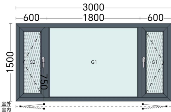
办公室大样参考图1
