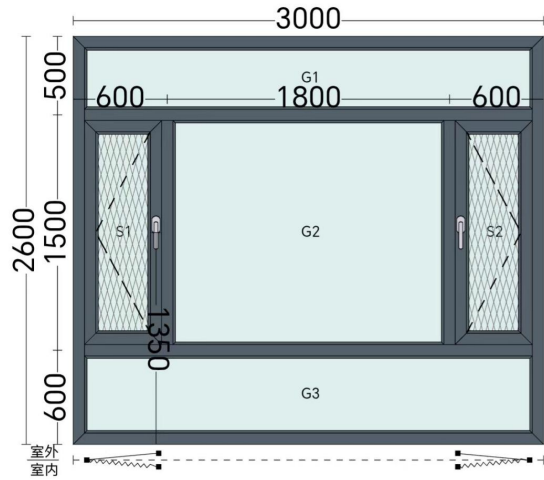
二层实验室大样参考图4
